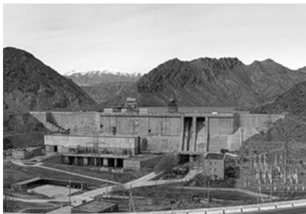
Рисунок 2.55. Таш-Кумырская ГЭС
