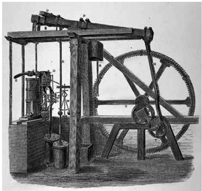
Рисунок 3.3. Паровая машина Джеймса Уатта
