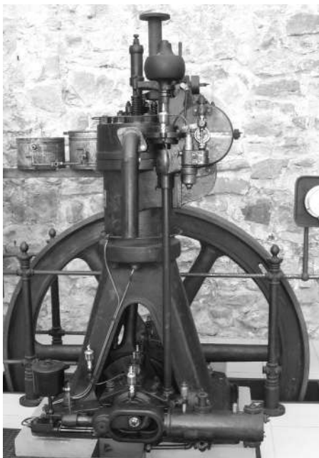
Рисунок 3.2. Двигатель Рудольфа Дизеля
