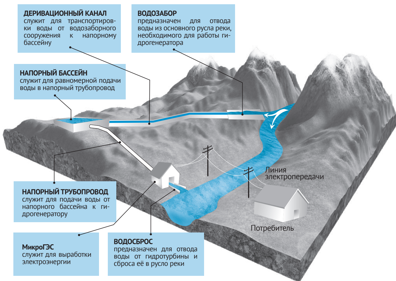
Рисунок 2.57. Принцип действия малой ГЭС 2
