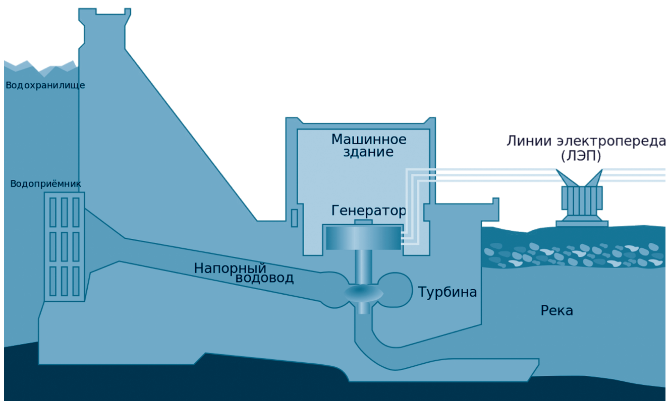
Рисунок 2.52. Устройство работы ГЭС
