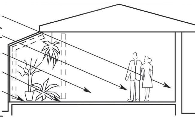
Рисунок 2.30. Пассивное отопление дома с использованием оранжереи
