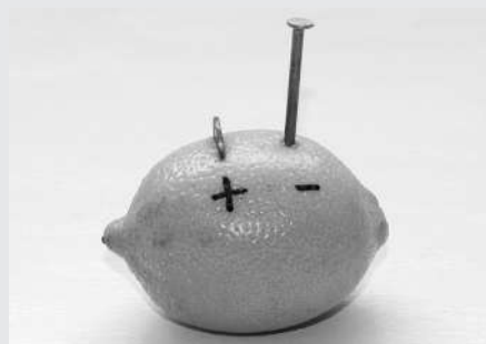
Рисунок 1.11. Оцинкованный винт, вкрученный в лимон
