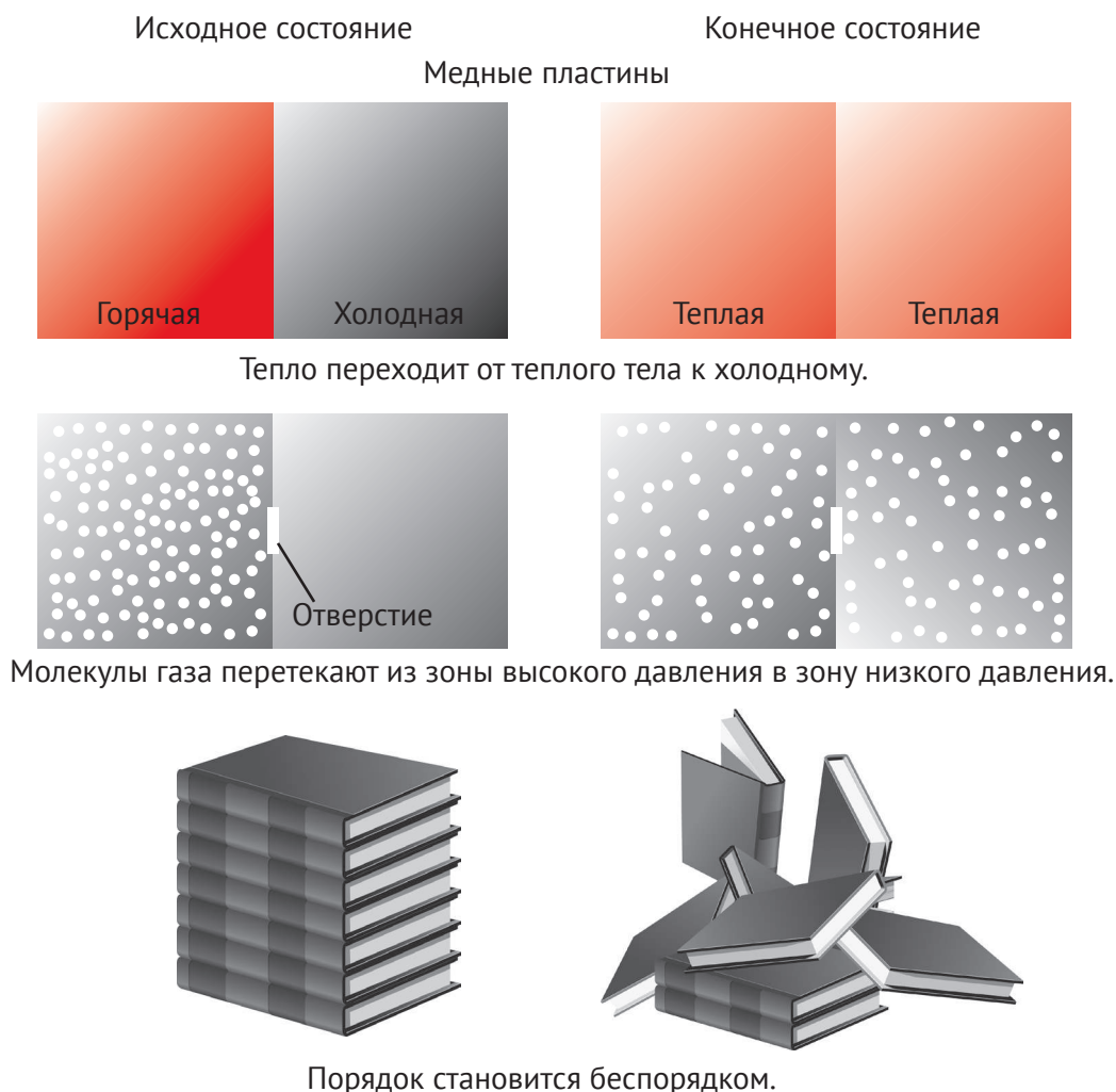
Рисунок 1.20. Иллюстрации второго закона термодинамики
