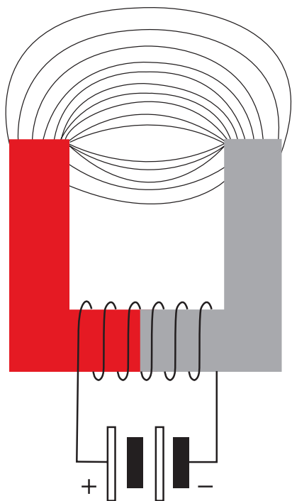
Рисунок 1.10. Образование электромагнитной энергии
