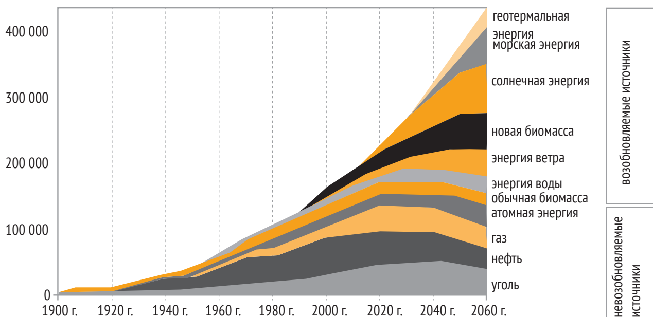
Рисунок 3.6. Структура потребления энергии в мире по источникам с прогнозом до 2060 года
