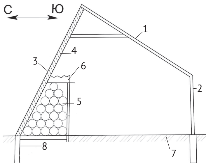
Рисунок 2.33. 1 – прозрачная изоляция, 2 – опорная стенка, 3 – северная стена, 4 – теплоизоляция, 5 – галечный аккумулятор, 6 – ящики с рассадой, 7 – защищенный грунт, 8 – теплоизолированный фундамент.
