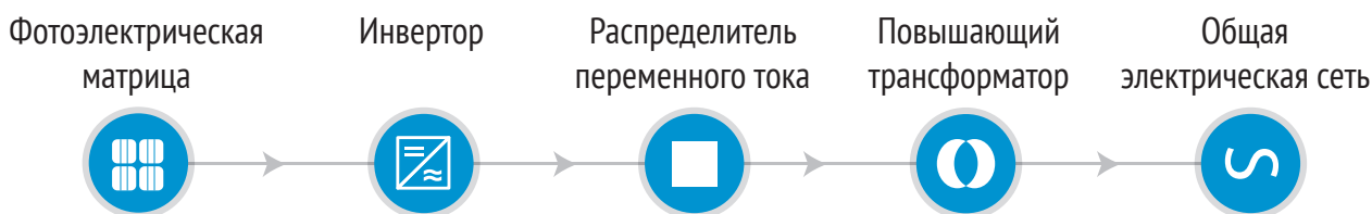
Рисунок 2.36. Схема преобразования постоянного тока в переменный ток гелиостанцией, включенной в электросеть
