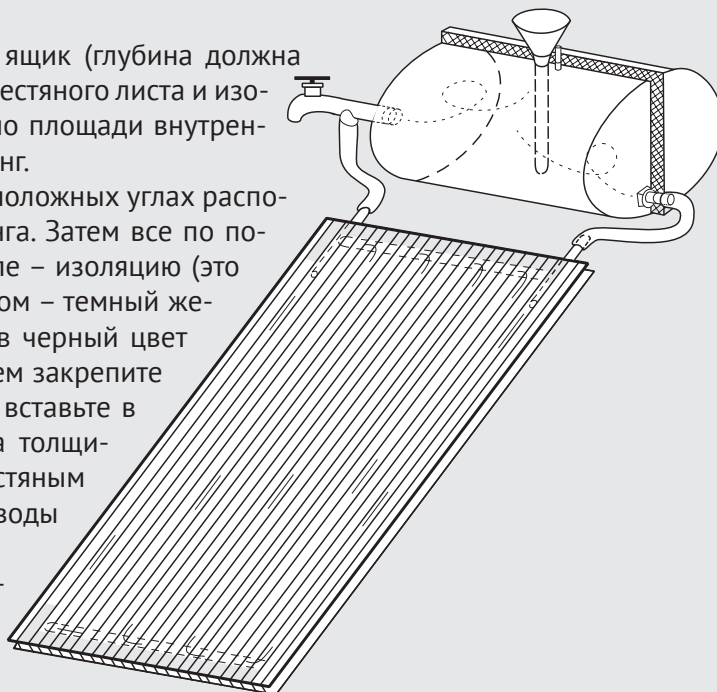
Рисунок 2.21. Схема солнечного коллектора
