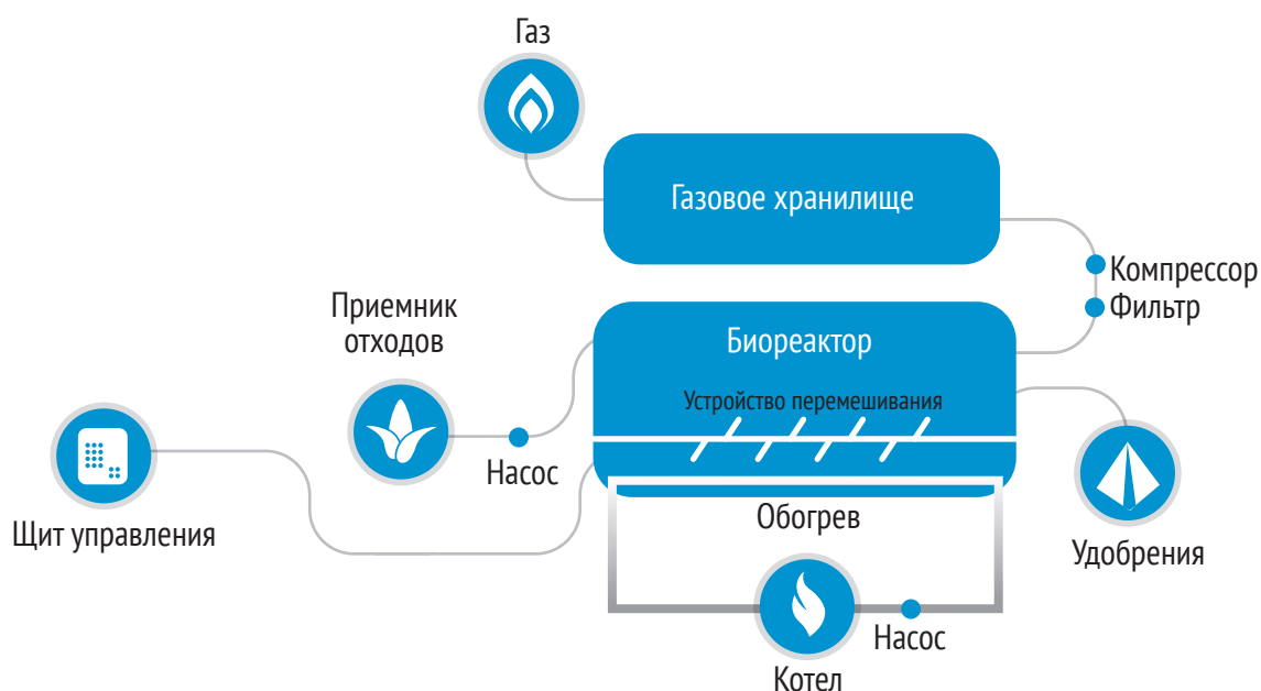
Рисунок 2.43. Схема устройства биогазовой установки
