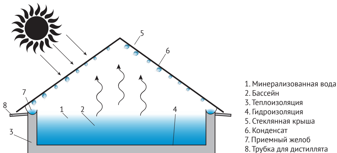
Рисунок 2.15. Солнечный дистиллятор-бассейн
