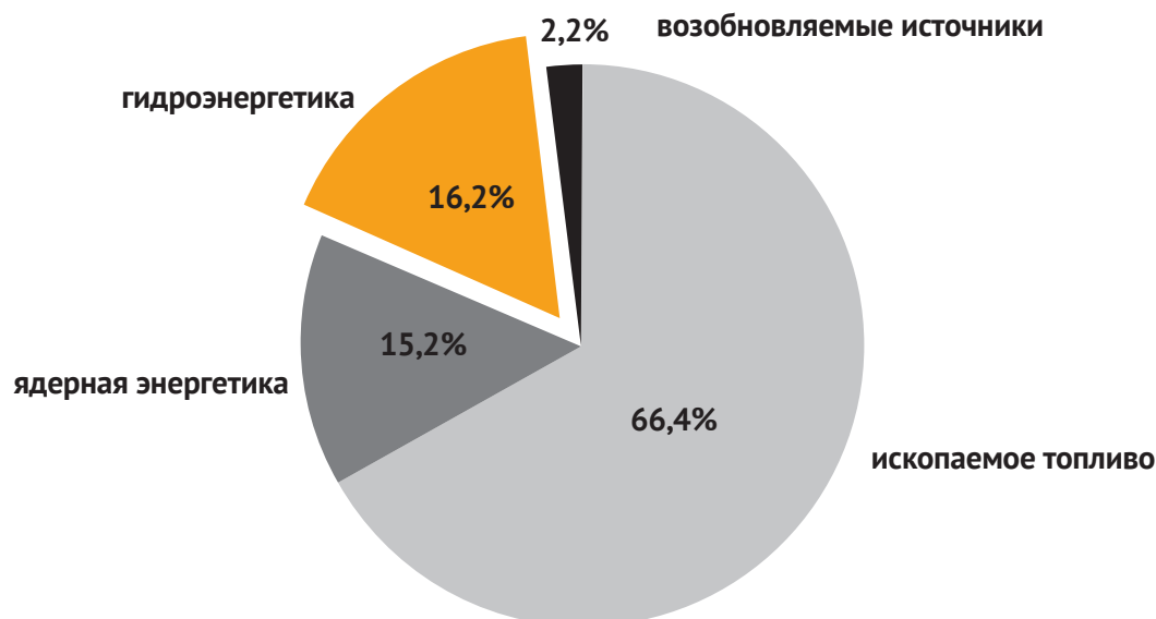
Рисунок 3.7. Мировое потребление энергии от различных источников
