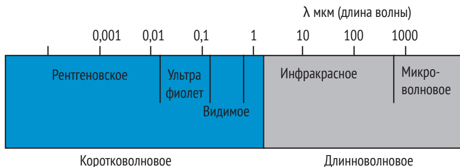
Рисунок 2.14. Волновой диапазон солнечного излучения
