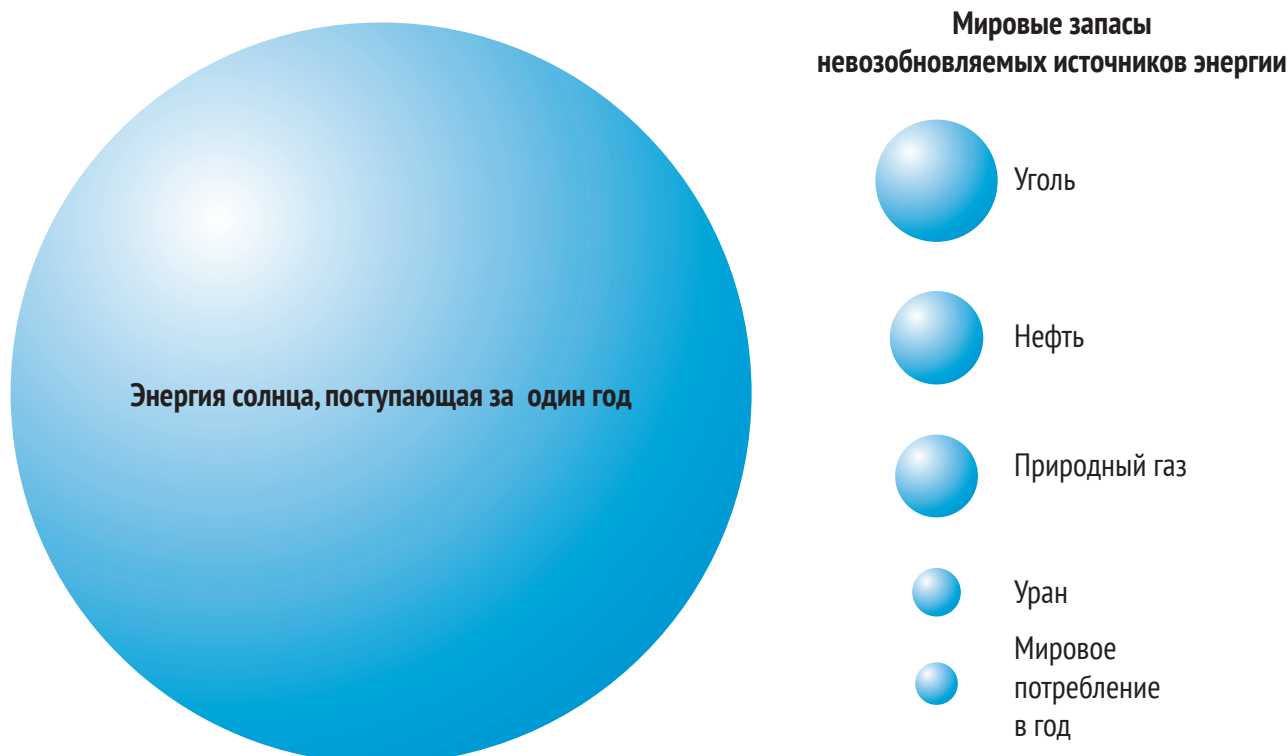
Рисунок 2.2. Годовой приход солнечной энергии в сравнении с запасами невозобновляемых источников энергии
