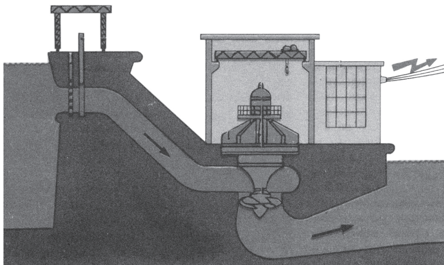
Рисунок 1.16. Плотина гидроэлектростанции. Вода, падая с высоты, теряет потенциальную энергию и приобретает кинетическую 1 .
