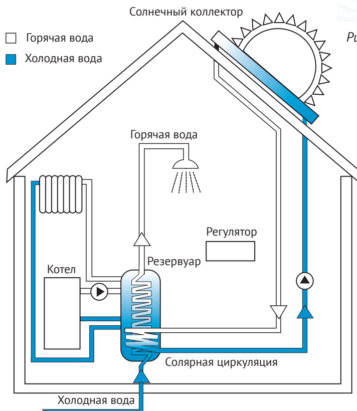
Рисунок 2.32. Система отопления с использованием солнечных коллекторов
